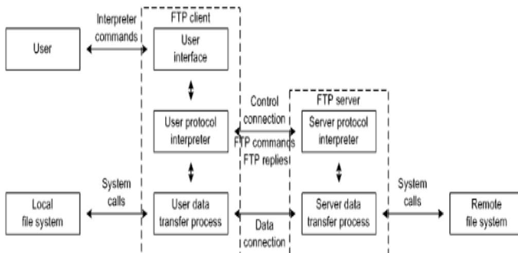
Структура FTP-системы
